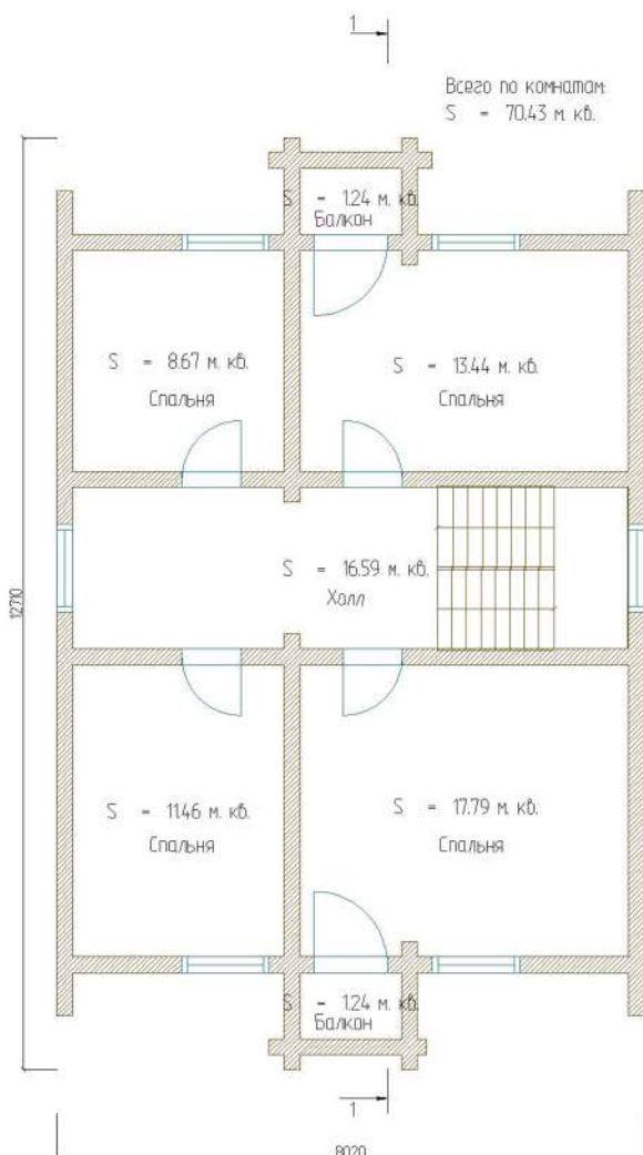
План 2го этажа
